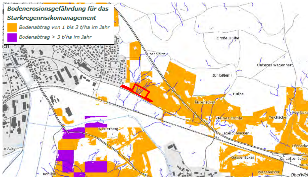
Abbildung 10: Bodenerosionsgefährdung mit Abflussbahnen (blaue Linien) für das Starkregenrisikomanagement, Lage des Plangebietes rot umrandet. Quelle: LGRB Kartenviewer online, abgerufen am 23.02.2022.
