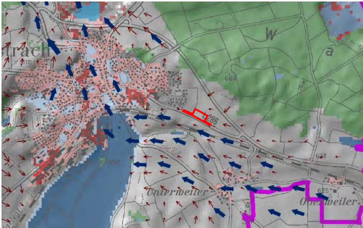
Abbildung 12: Klimaanalysekarte des Regionalverbandes Bodensee-Oberschwaben. Plangebiet rot umrandet, unmaßstäblich.
